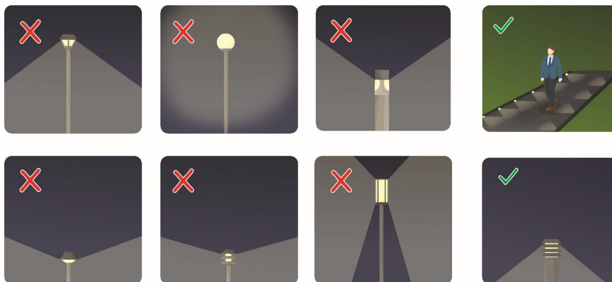
Figure 12 L'éclairage des allées doit être monté aussi bas que possible et protégé. Figure adaptée de Witherington et Martin (2003).
