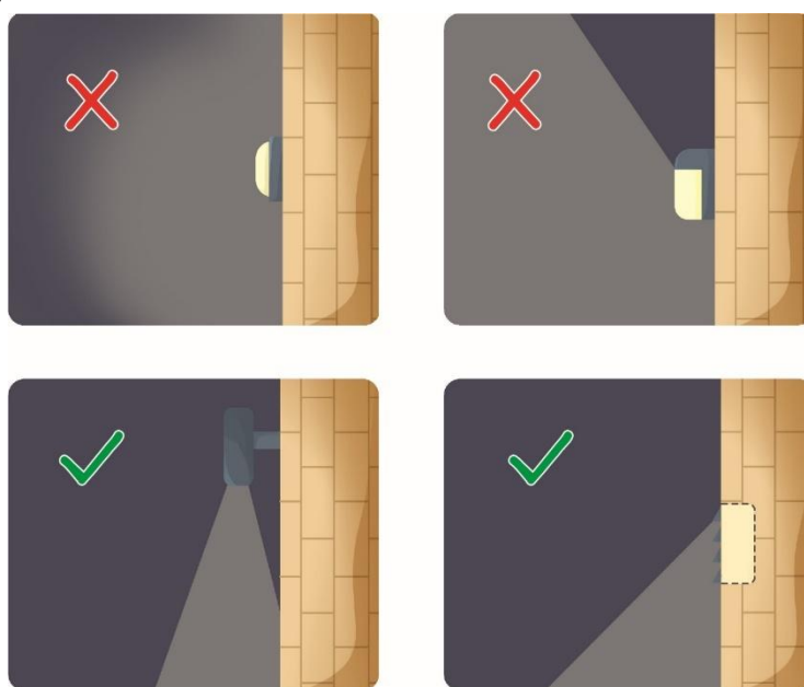
Figure 13 L'éclairage doit être dirigé de sorte à s'assurer que seule la zone prévue est éclairée. Figure adaptée de Witherington et Martin (2003).
