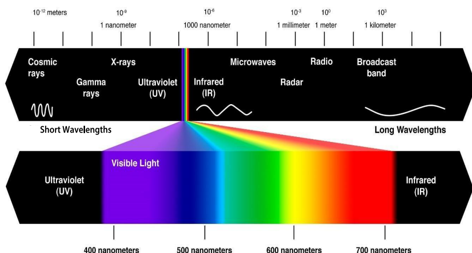
Figure 16 Le spectre électromagnétique. Le « spectre de la lumière visible » se situe entre 380 et 780 nm et constitue la partie du spectre que l'œil humain peut voir. Crédit : Mihail Pernichev (Iristech, 2018).
