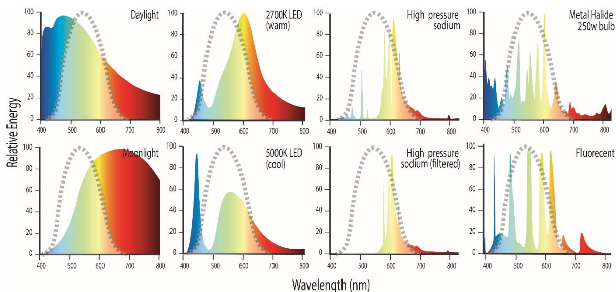
Figure 26 Les instruments photométriques ne quantifient que la lumière située à l'intérieur de la courbe CIE (zone située sous la ligne pointillée grise). Ces résultats sont comparés aux courbes spectrales d'une série de sources lumineuses différentes.
