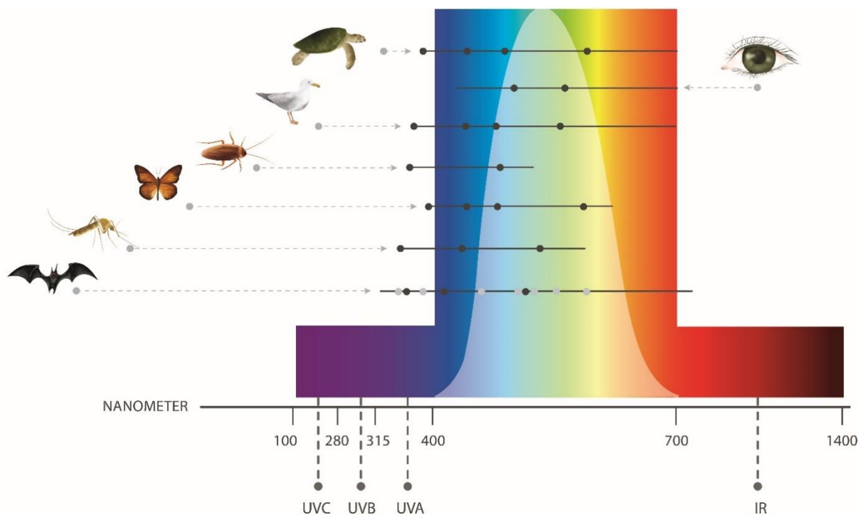
Figure 2 Capacité à percevoir différentes longueurs d'onde de lumière chez l'homme et la faune montré par les lignes horizontales. Les points noirs représentent les pics de sensibilité signalés. Les points noirs pour les chauves-souris représentent les pics de sensibilité chez une chauve-souris omnivore, d'après Winter et autres (2003) ; les points gris représentent les pics de sensibilité potentiels chez les chauves-souris, tirés de Feller et autres (2009) et Simões et autres (2018). Figure adaptée de Campos (2017).
