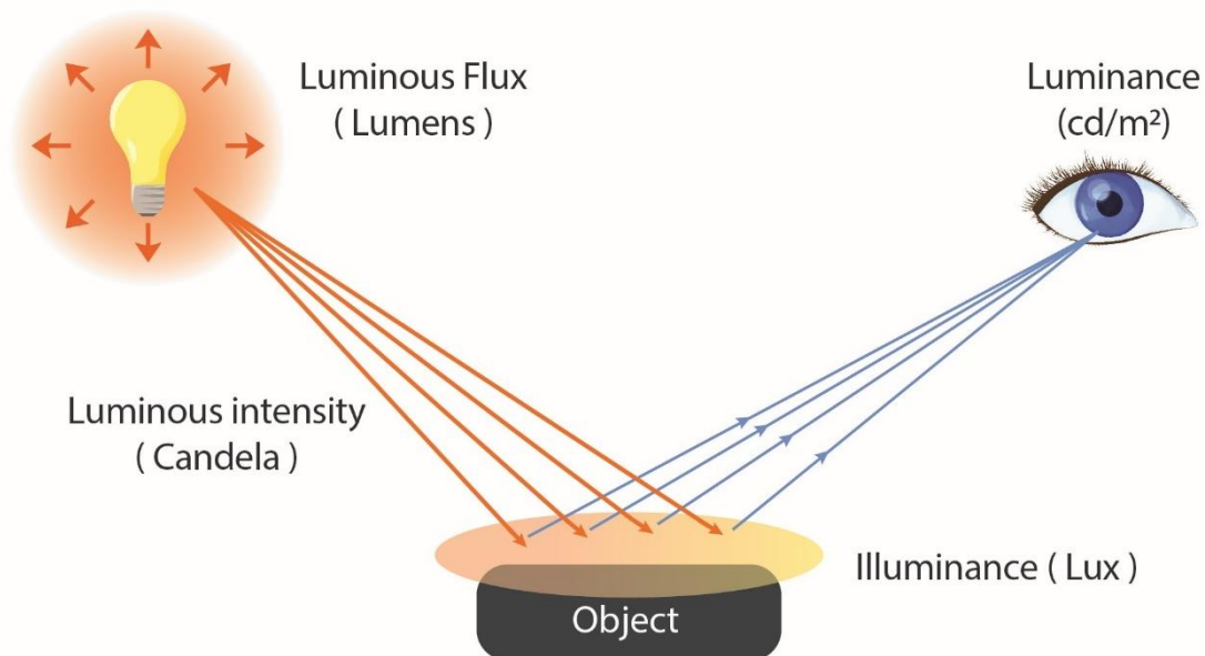
Figure 19 Flux lumineux, luminance et éclairage.
