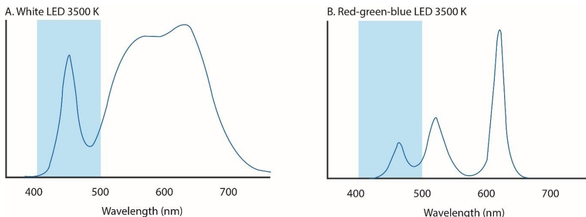
Figure 24 Comparaison du contenu spectral de la longueur d'onde bleue de deux lampes LED ayant le même TCC (3 500 K). La bande bleue représente la région bleue du spectre visible (400-500 nm). La lumière de A a une teneur en lumière bleue beaucoup plus importante que celle de B, mais l'œil humain a l'impression qu'il s'agit de la même couleur. Pour les animaux dont la sensibilité à la longueur d'onde de la lumière diffère de celle de l'homme, elles peuvent apparaître très différentes. Figure reproduite avec l'aimable autorisation de Ian Ashdown.
