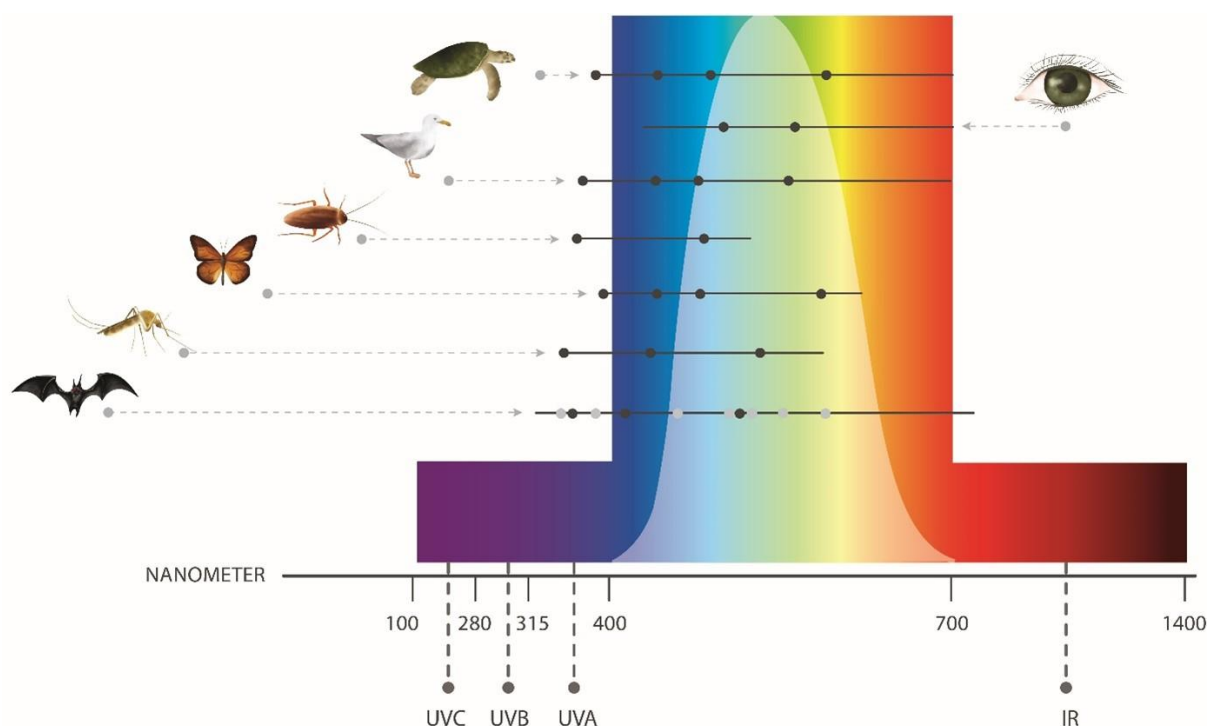
Figure 22 Lumière photométrique représentée par l'aire sous la courbe CIE (aire blanche) comparée à la capacité de percevoir différentes longueurs d'onde (lignes noires) et à la sensibilité maximale déclarée (points noirs) chez l'homme et la faune. Noter que la zone sous la courbe CIE n'inclut pas une grande partie de la lumière violette et ultraviolette visible par de nombreux animaux. Figure adaptée de Campos (2017).
