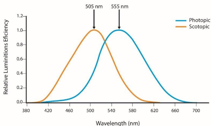
Figure 18 Fonctions de luminosité scotopique et photopique chez l'homme. Source de données : Fonctions de luminosité .
