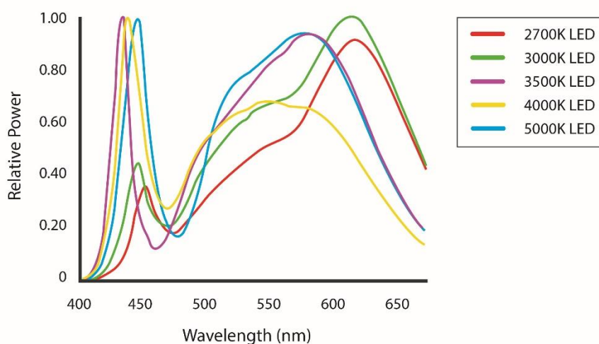
Figure 23 Courbes spectrales montrant la teneur en bleu des lumières LED blanches de 2 700 à 5 000 K. Noter la différence de puissance relative dans la gamme des longueurs d'onde bleues (400 – 500 nm). Figure reproduite avec l'aimable autorisation de Ian Ashdown.
