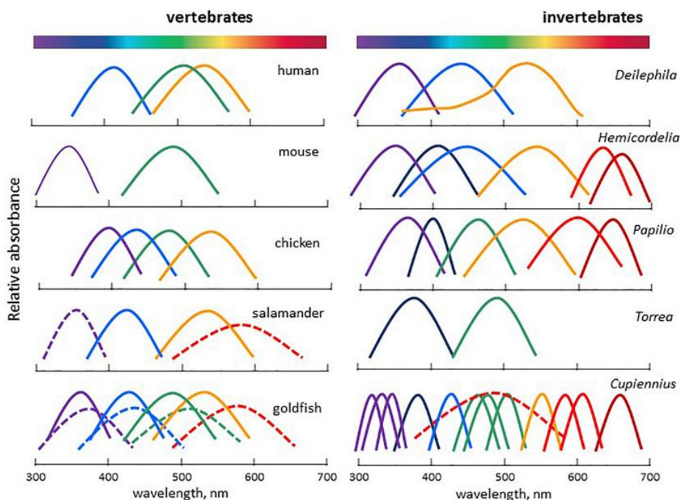
Figure 17 Capacité à percevoir différentes longueurs d'onde de la lumière chez l'homme et les espèces animales. Figure tirée de Falcón et autres (2020), adaptée et modifiée à partir de Imamoto et Shichida (2014), Warrant (2019).
