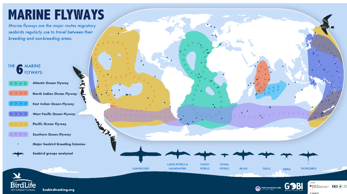
Figure 4.3 : Les six voies migratoires marines à travers les océans du monde, illustrant les migrations récurrentes des oiseaux de mer pélagiques. Crédit image : BirdLife International.
