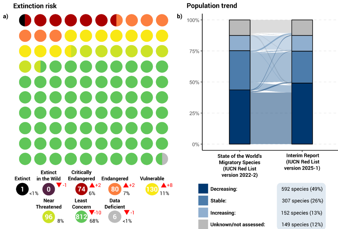
Figure 1.1 : a) Proportion et nombre d'espèces inscrites aux Annexes de la CMS dans chaque catégorie de la Liste rouge de l'UICN. Dans le graphique principal, chaque cercle représente 1 % des 1 200 espèces inscrites aux Annexes de la CMS. La légende ci-dessous indique le nombre total d'espèces inscrites aux Annexes de la CMS actuellement dans chaque catégorie. Les chiffres et flèches rouges indiquent le changement net entre le Rapport sur l'état des espèces migratrices dans le monde et le présent rapport*. Les changements nets excluent les espèces inscrites lors de la COP14 ainsi que les espèces inscrites au niveau des populations pour lesquelles des évaluations pertinentes à l'échelle régionale sont devenues disponibles depuis le Rapport sur l'état des espèces migratrices dans le monde . Les changements nets peuvent refléter à la fois des détériorations ou améliorations de l'état de conservation liées à l'intensification ou la réduction des menaces, ou des modifications de catégorie résultant d'une meilleure connaissance des données. b) Évolution des tendances des populations des espèces inscrites aux Annexes de la CMS entre le Rapport sur l'état des espèces migratrices dans le monde et le présent rapport* . La légende indique le nombre total d'espèces inscrites aux Annexes de la CMS dans chaque catégorie de tendance des populations ; les taxons ajoutés aux Annexes de la CMS lors de la COP14 sont exclus du graphique.
