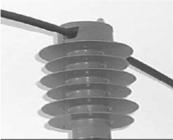
Figure 6. Exemple d'un câble isolé (câble noir), utilisé en Hongrie (source : Podonyi, 2011).
